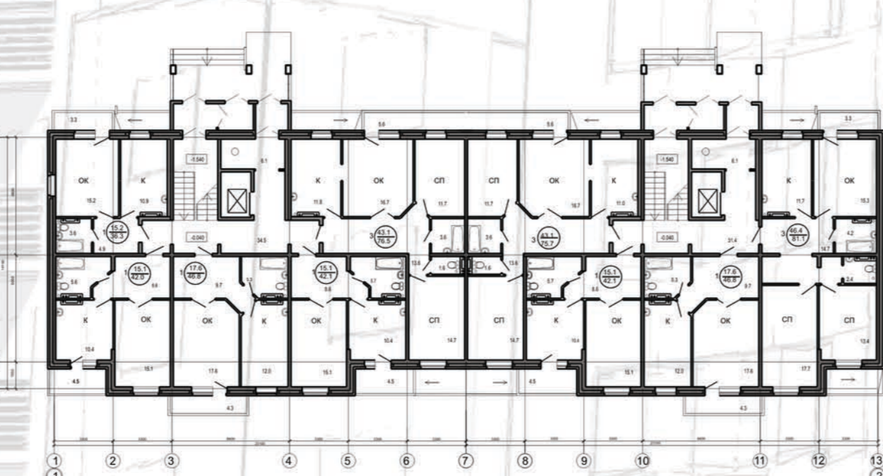
Блок-секция 1-2 1 этаж
