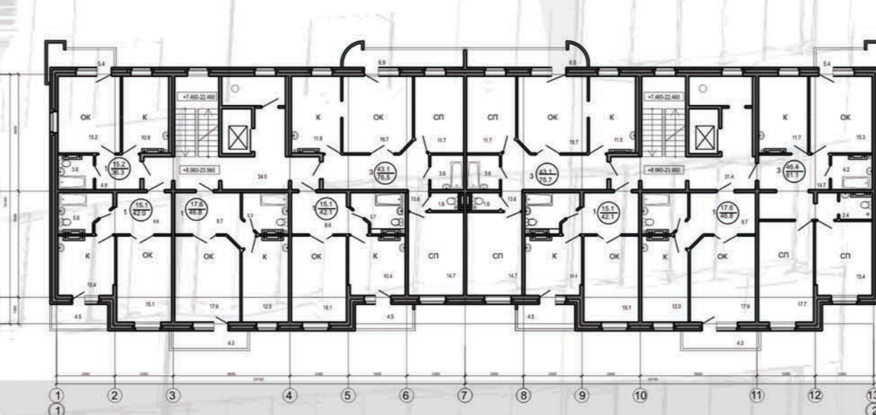
Блок-секция 1-2 типовой этаж
