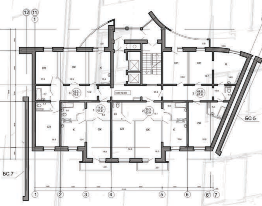
Блок-секция 6 типовой этаж.
