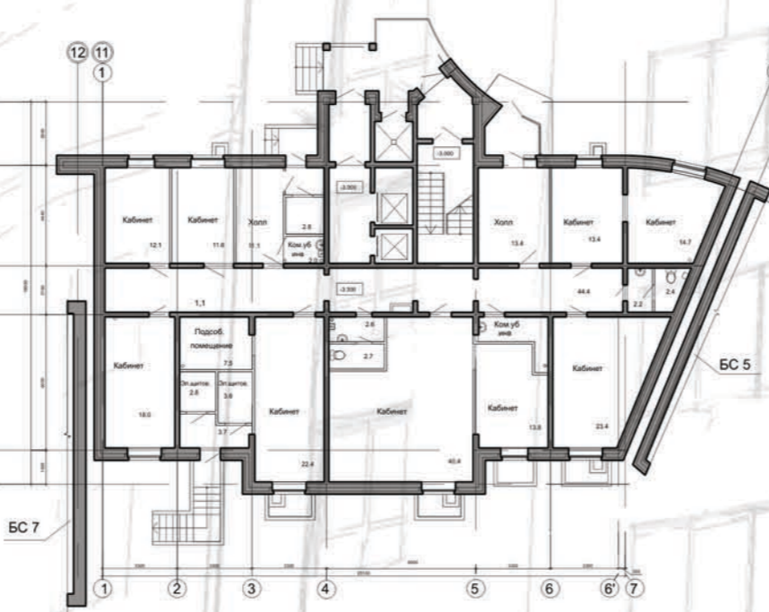
Блок-секция 6 1 этаж.
