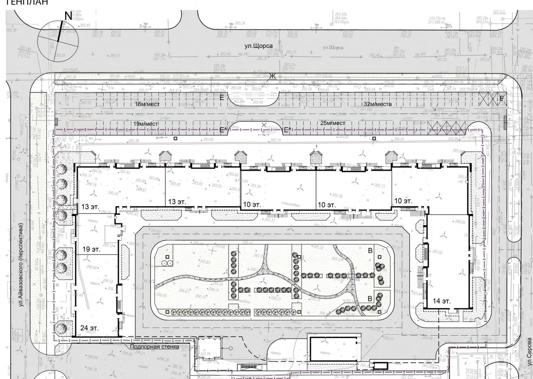
ГЕНПЛАН
