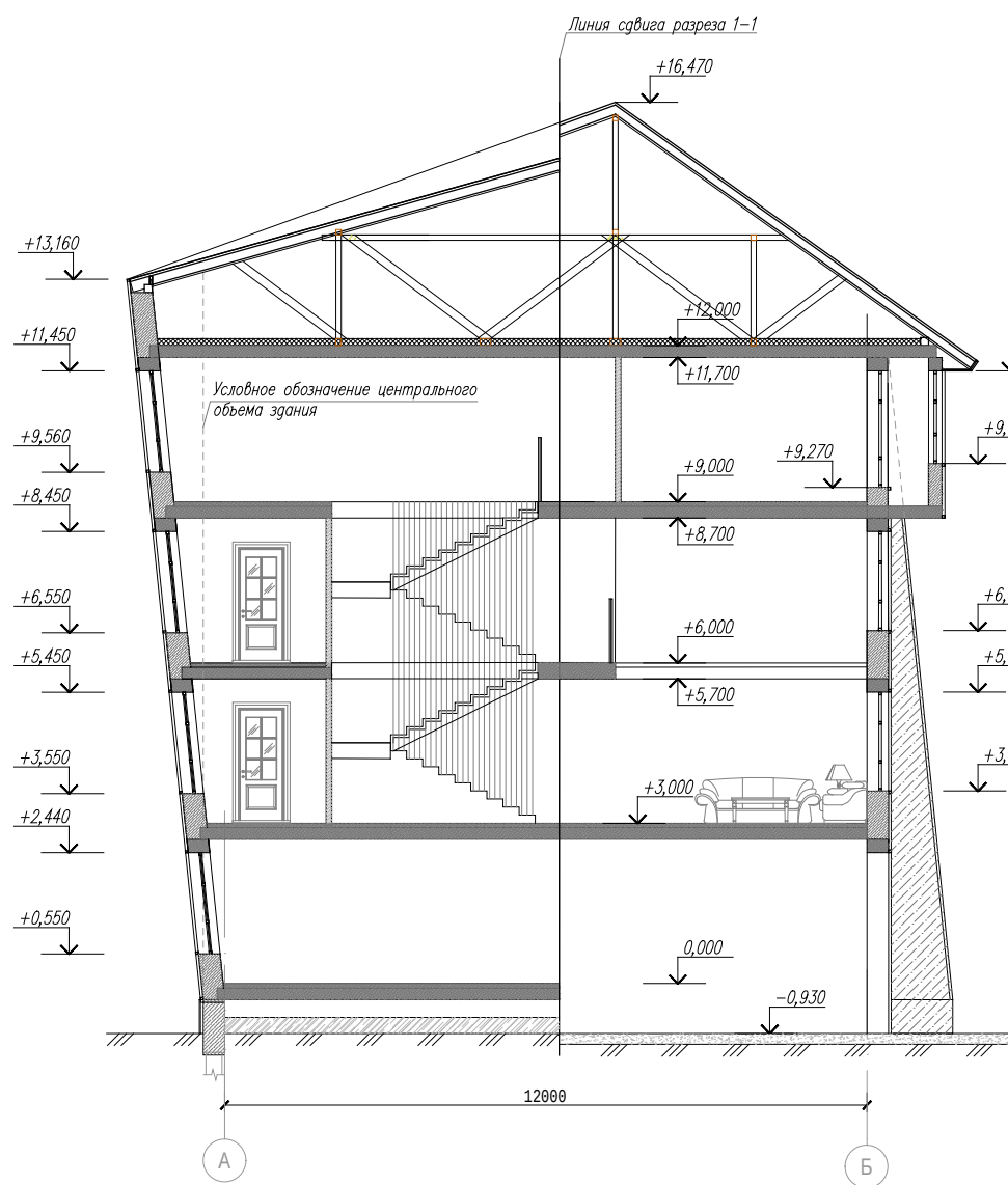
Разрез 1-1
