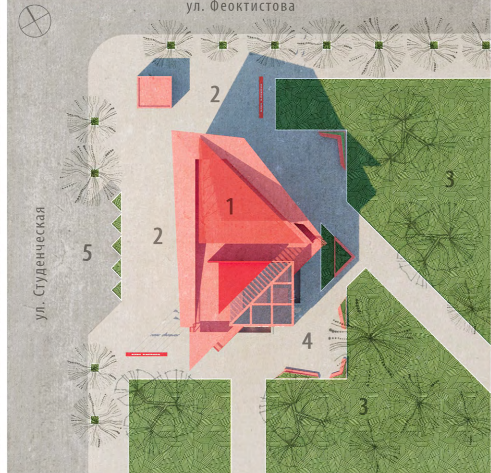
Ситуационная схема Генеральный план
