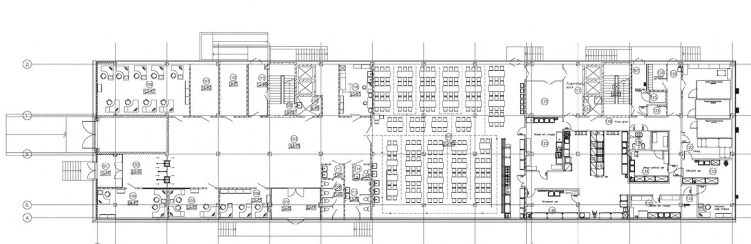
КОРПУС D. ПЛАН 1 ЭТАЖА
