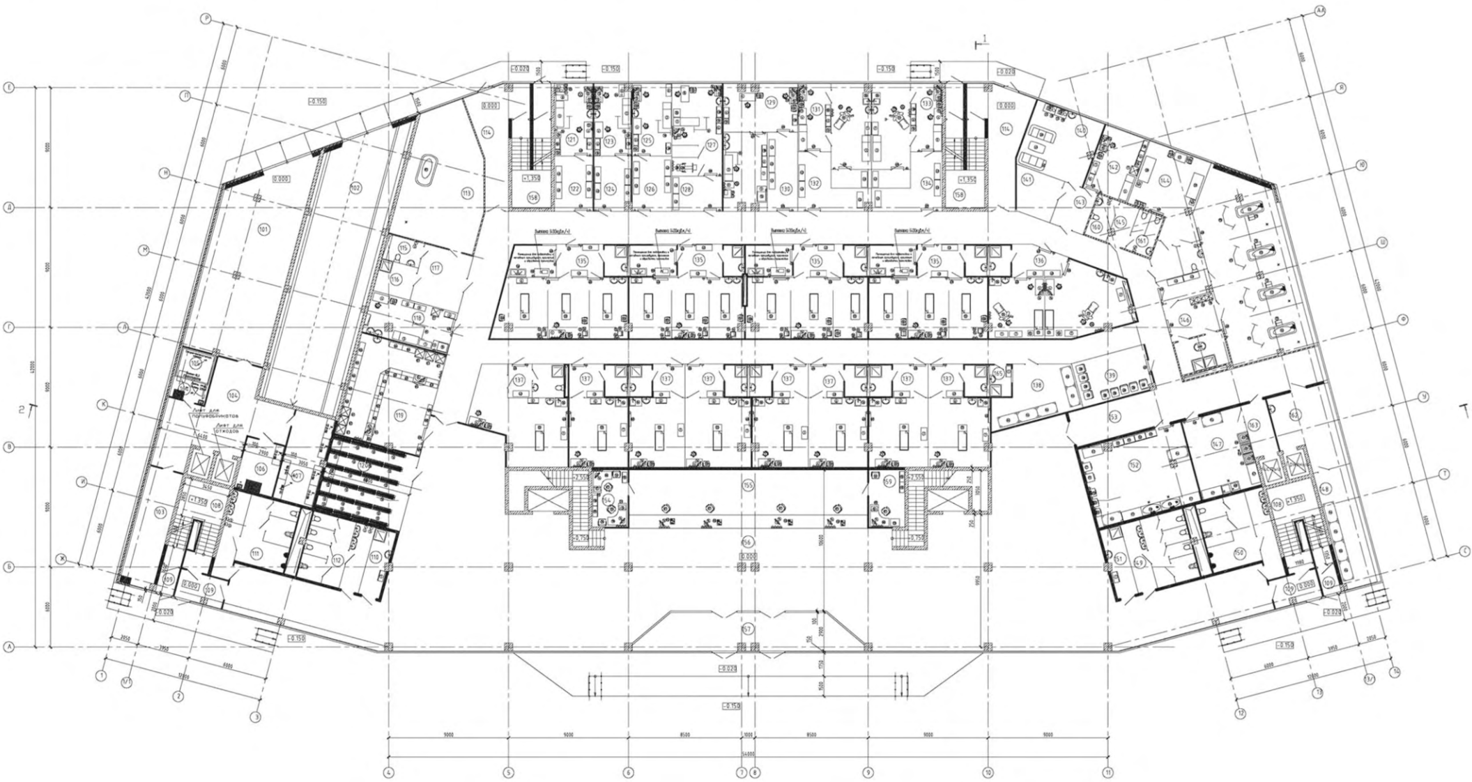
КОРПУС В2. ПЛАН 1 ЭТАЖА
