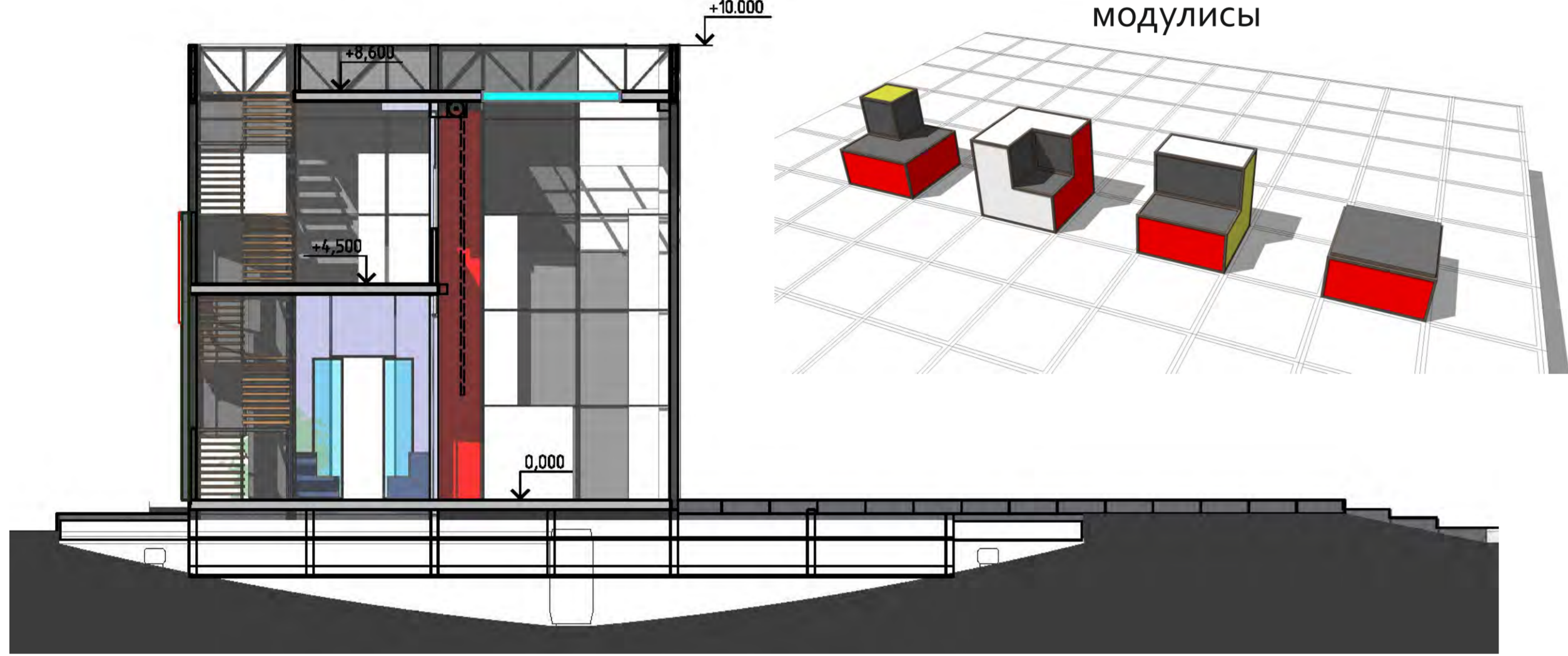
Продольный разрез
