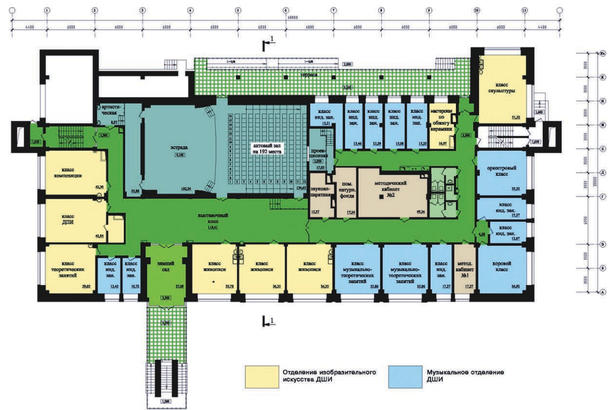
План 2-ого этажа
