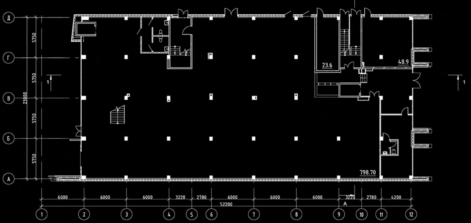
ПЛАН 2 ЭТАЖА
