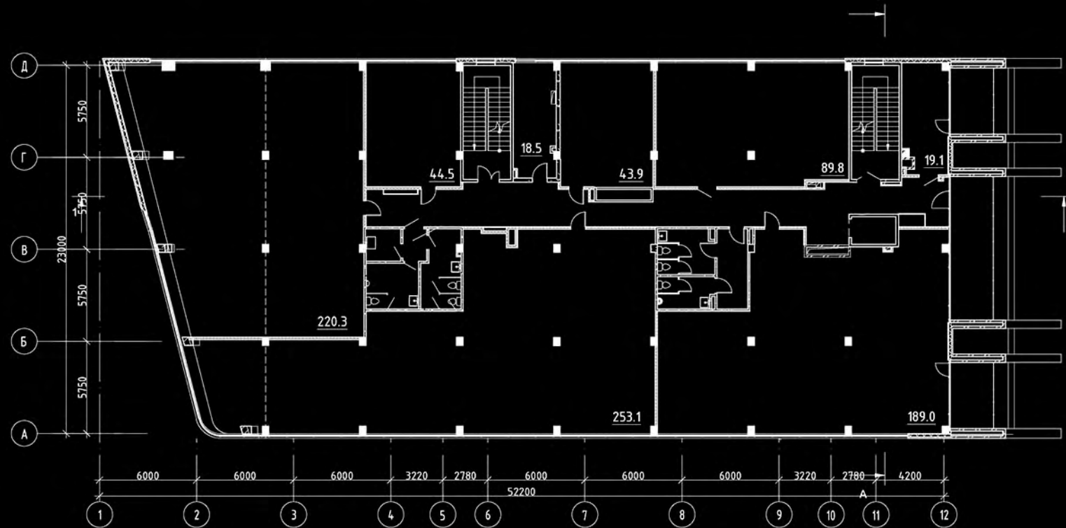
ПЛАН 2 ЭТАЖА
