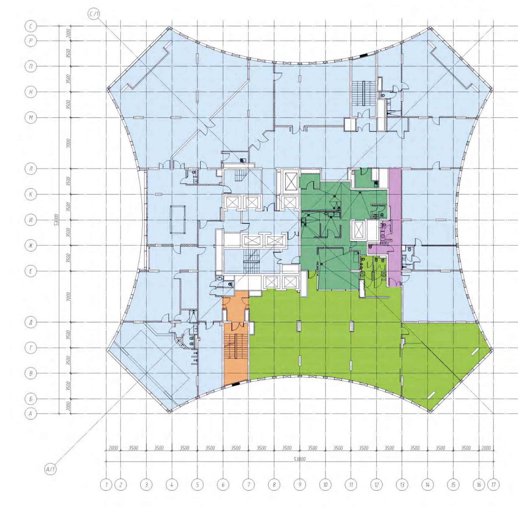
ПЛАН 14-ого ЭТАЖА
