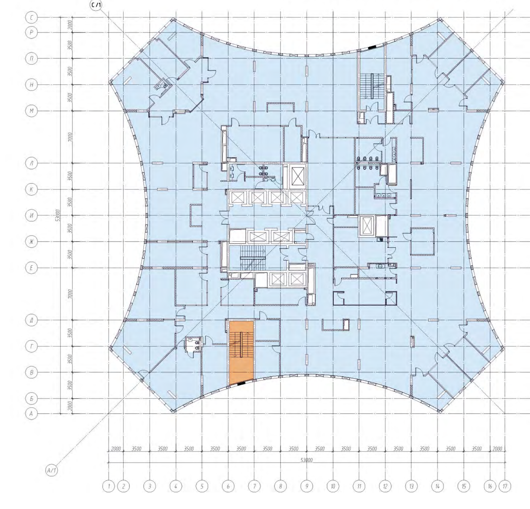
ПЛАН ТИПОВОГО ЭТАЖА (10-13эт.)
